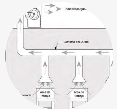
Campanas extracción
